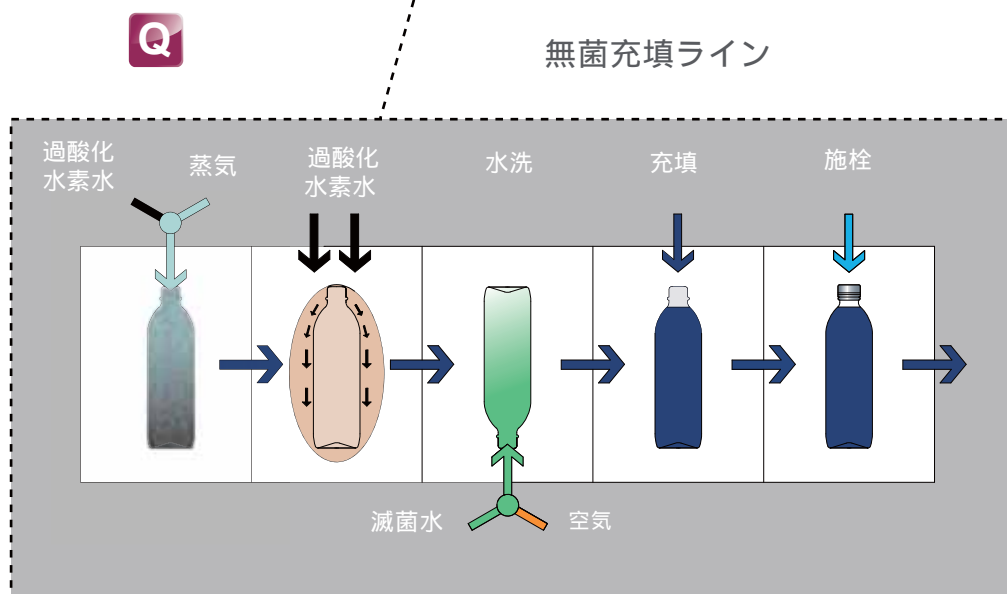
無菌充填プロセスの内部
