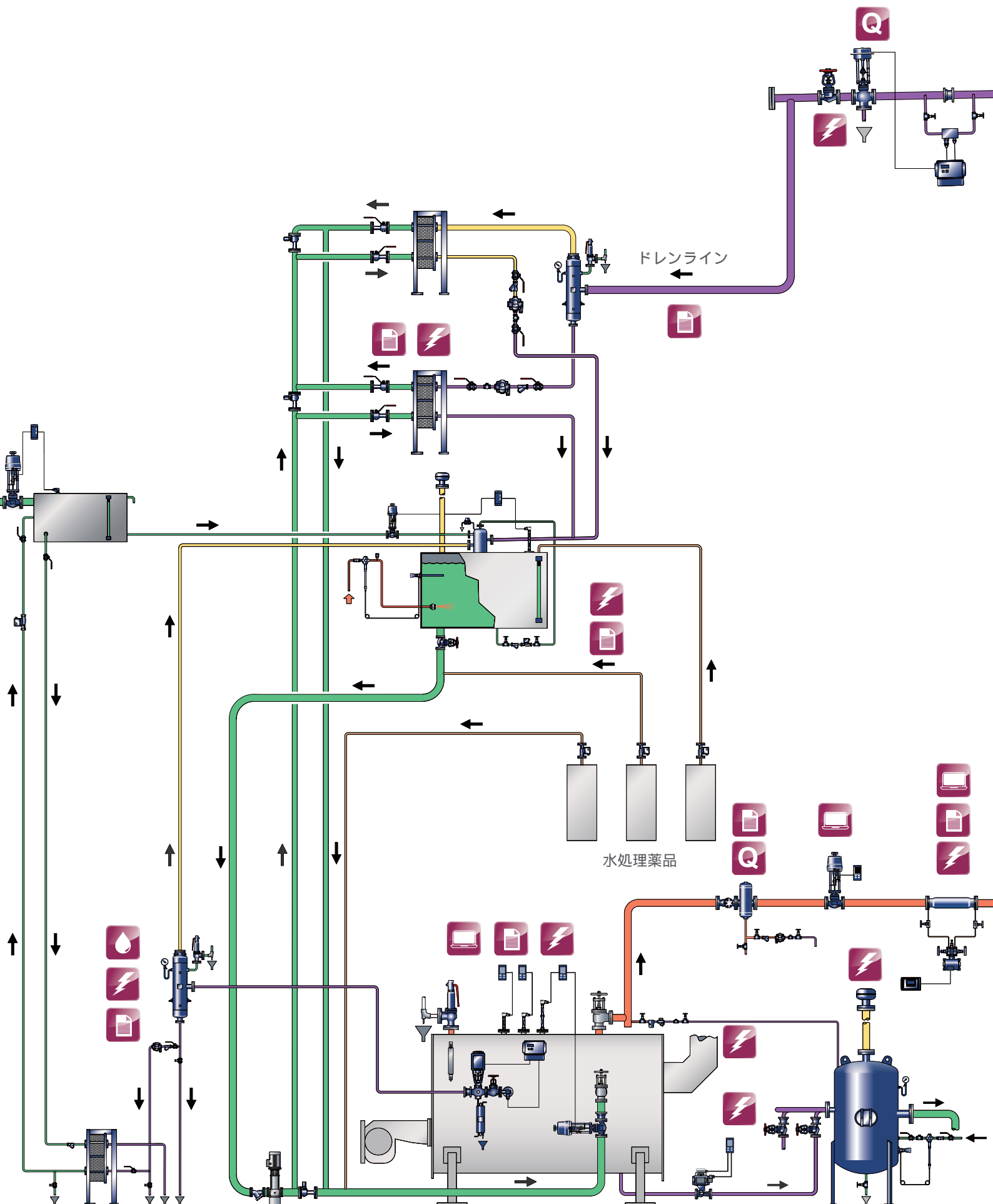
ボイラー室
